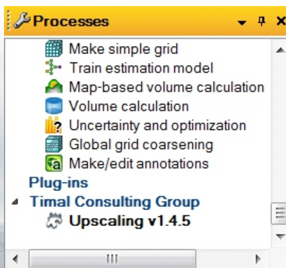
Рисунок 4 – Расположение плагина
