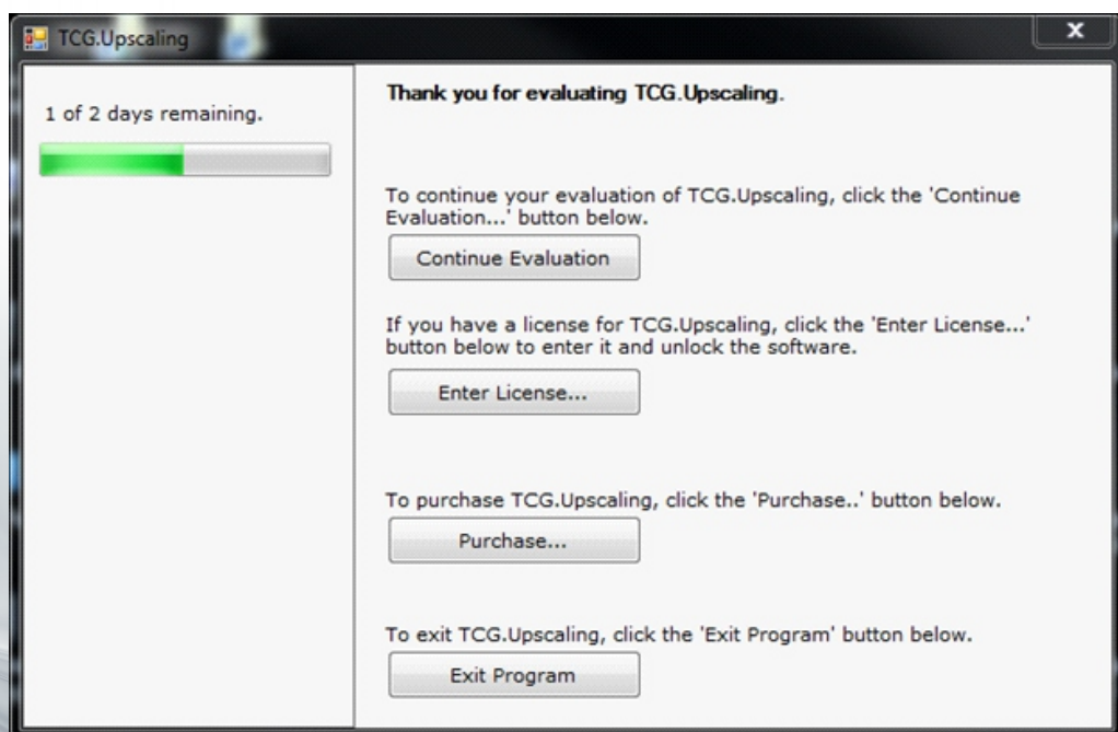
Рисунок 9 – Окно-напоминание
