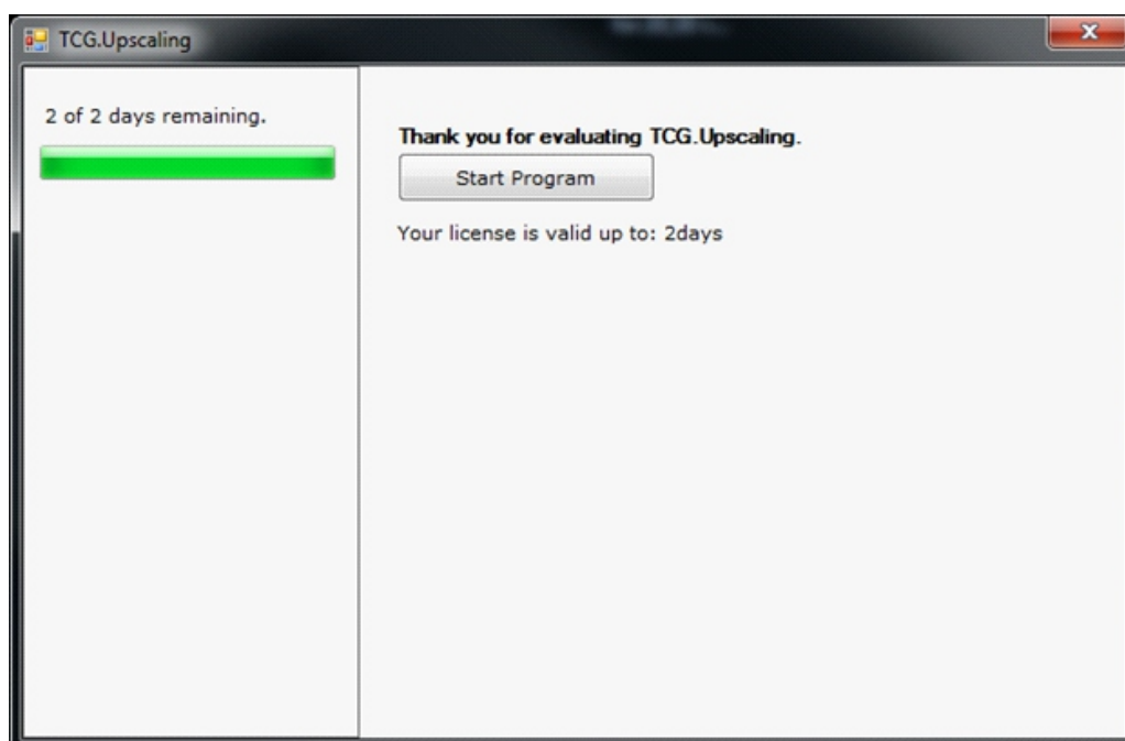
Рисунок 8 – Окно-приветствие
